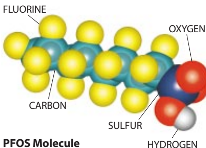
PFOS Molecule
